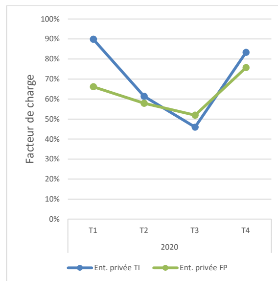
Figure 36: Facteur de charge des cogénérations ≤ 15 kWe en 2020 par type de titulaire
