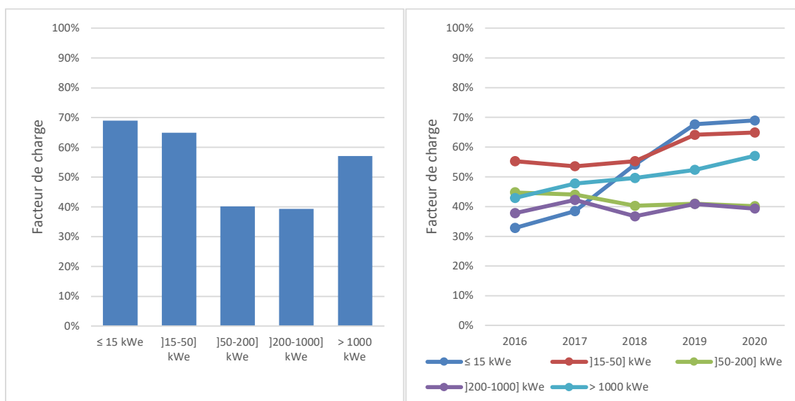
Figure 34: Facteur de charge annuel 2020 et évolution de 2016 à 2020, par catégorie de puissance
