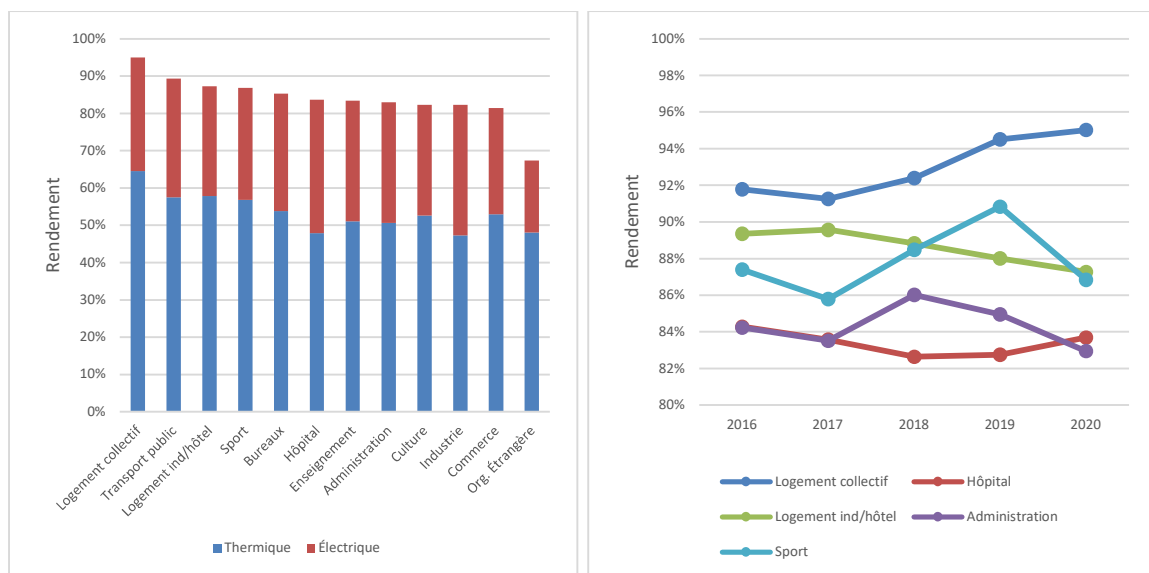
Figure 32: Rendement annuel 2020 et évolution de 2016 à 2020, par type de prosumer
