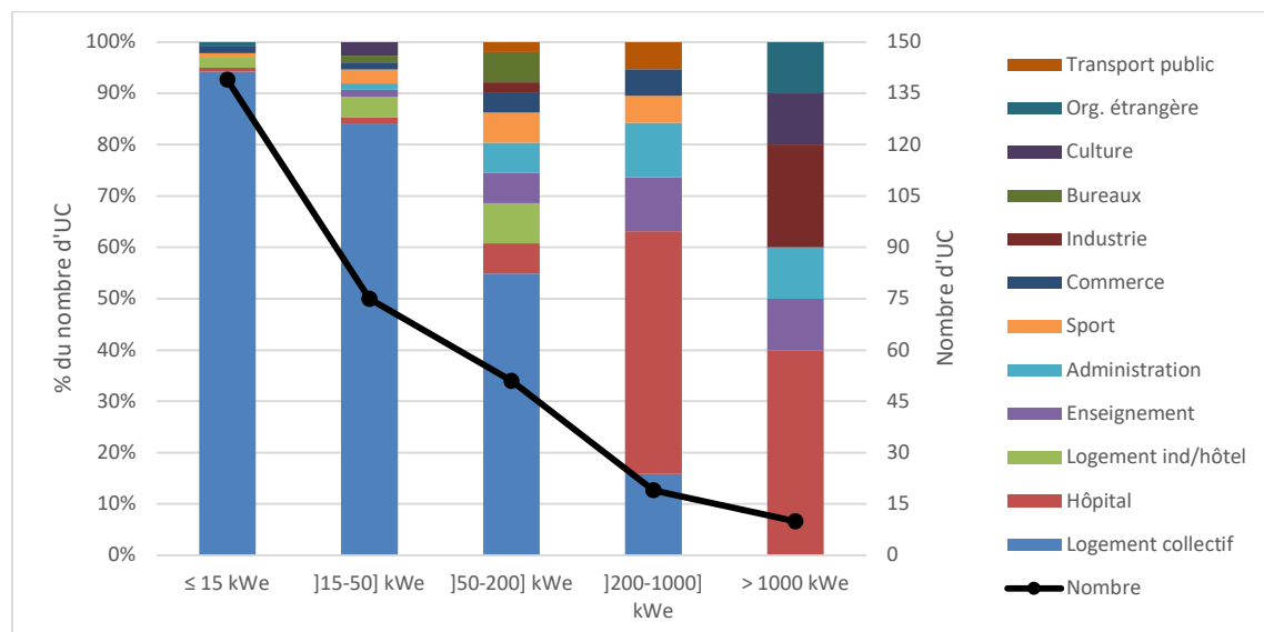
Figure 7: Nombre d'UC par catégorie de puissance ventilé par type de prosumer
