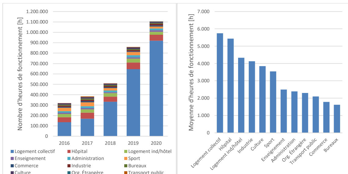
Figure 26: Nombre d'heures de 2016 à 2020 et moyenne annuelle 2020, par type de prosumer
