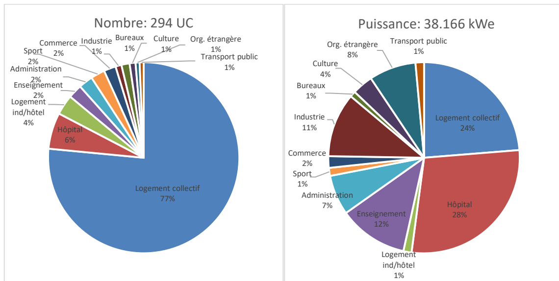
Figure 6: Nombre d'UC et puissance en service par type de prosumer
