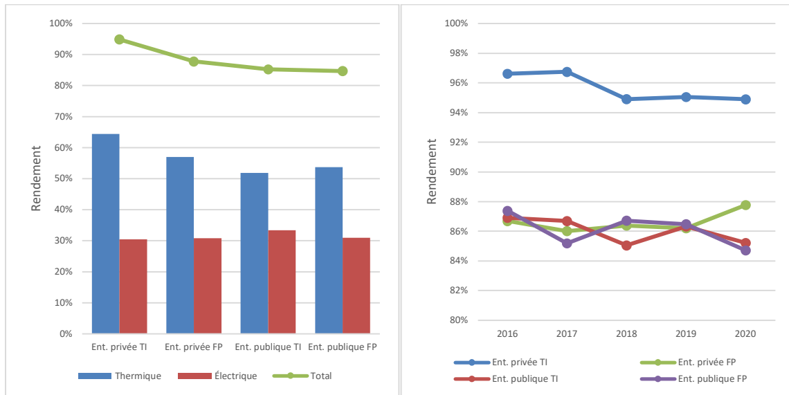
Figure 30: Rendement annuel 2020 et évolution de 2016 à 2020, par type de titulaire
