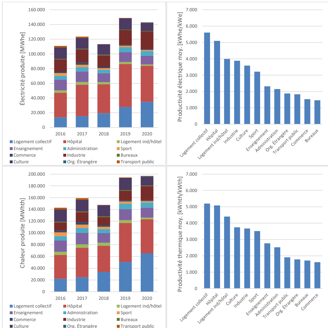
Figure 27: Production de 2016 à 2020 et productivité annuelle 2020, par type de prosumer
