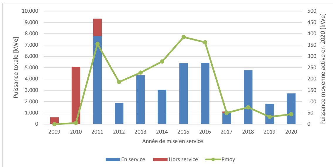
Figure 3: Puissance des UC actives en 2020 par année de mise en service
