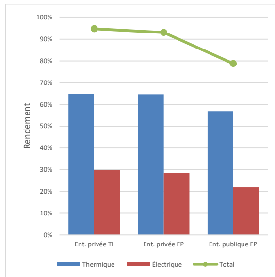
Figure 31: Rendement 2020 des installations ≤15 kWe par type de titulaire
