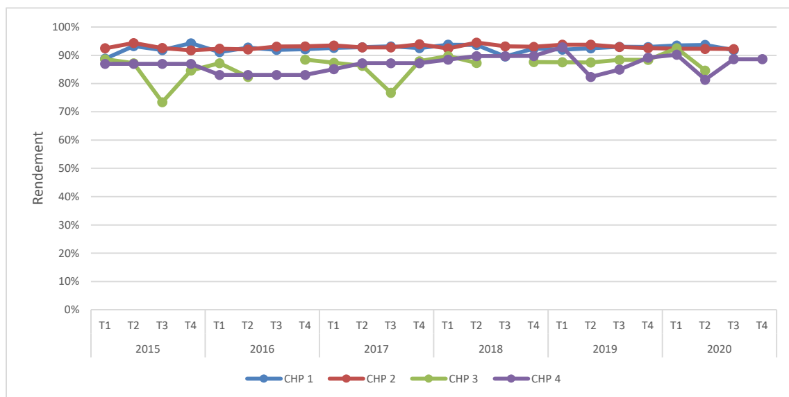
Figure 33: Évolution du rendement de 4 cogénérations mises en service en 2010
