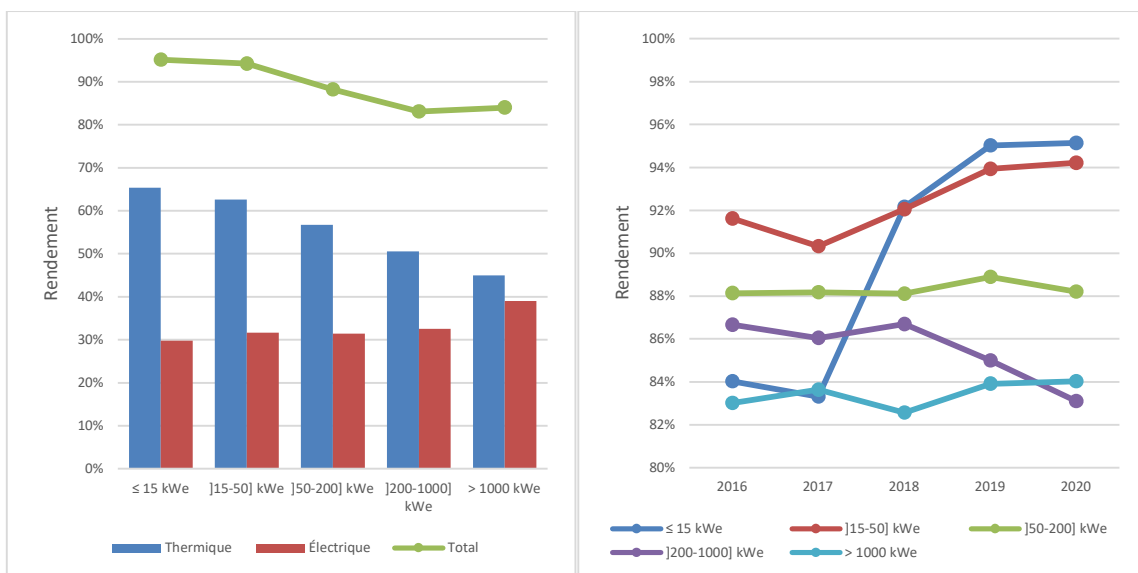
Figure 28: Rendement annuel 2020 et évolution de 2016 à 2020, par catégorie de puissance
